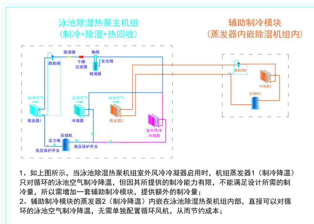
下图为除湿及辅助制冷系统流程图
