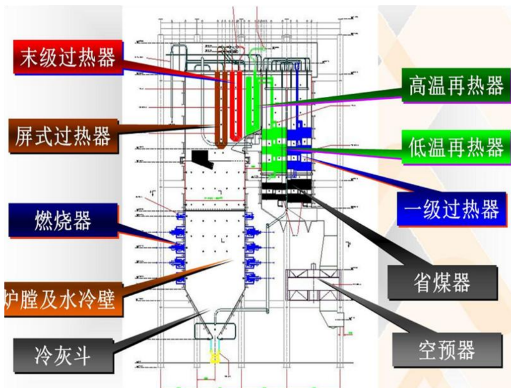
图 4 受热面布置示意图
