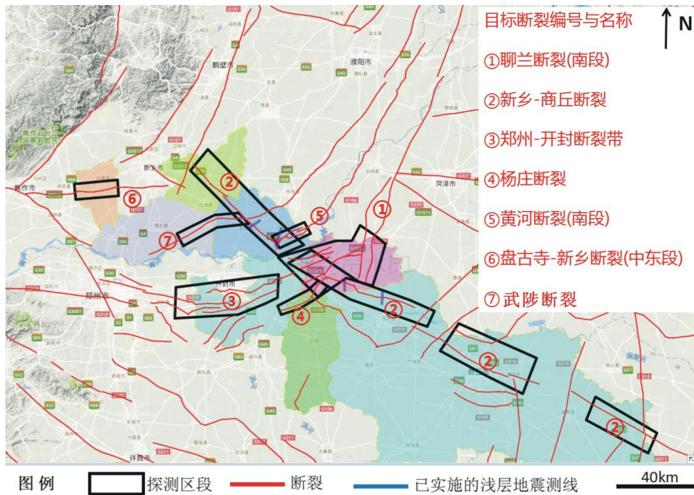
图 4-1 目标断裂与探测区段分布图
