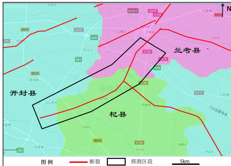
图 4-5 杨庄断裂探测区段分布图
