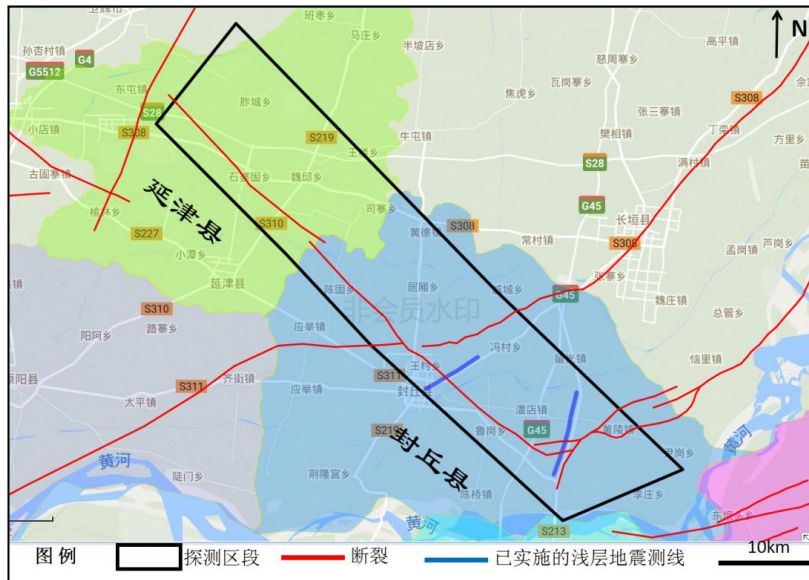
图 4-3A 新乡-商丘断裂延津-封丘段探测区段分布图
