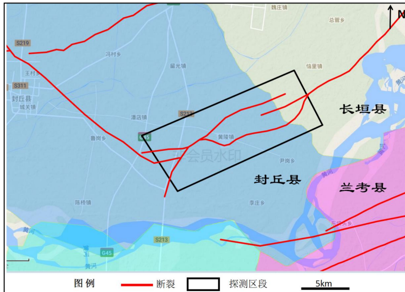
图 4-6 黄河断裂南段探测区段分布图
