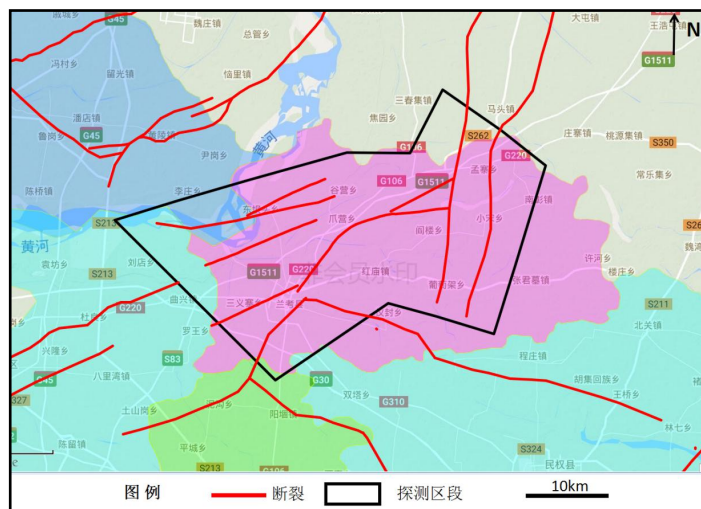
图 4-2 聊兰断裂南段探测区段分布图
