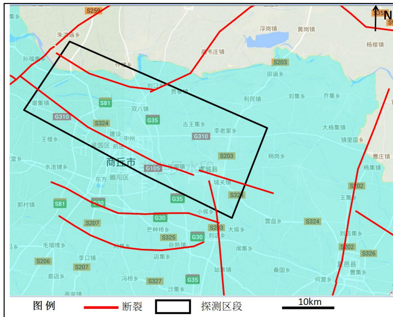
图 4-3C 新乡-商丘断裂商丘段探测区段分布图
