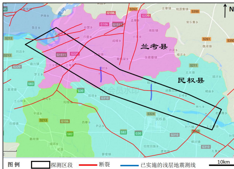
图 4-3B 新乡-商丘断裂兰考-民权段探测区段分布图
