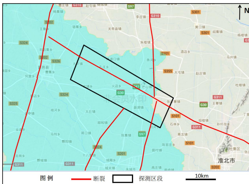
图 4-3D 新乡-商丘断裂永城段探测区段分布图
