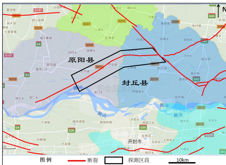
图 4-8 武陟断裂探测区段分布图
