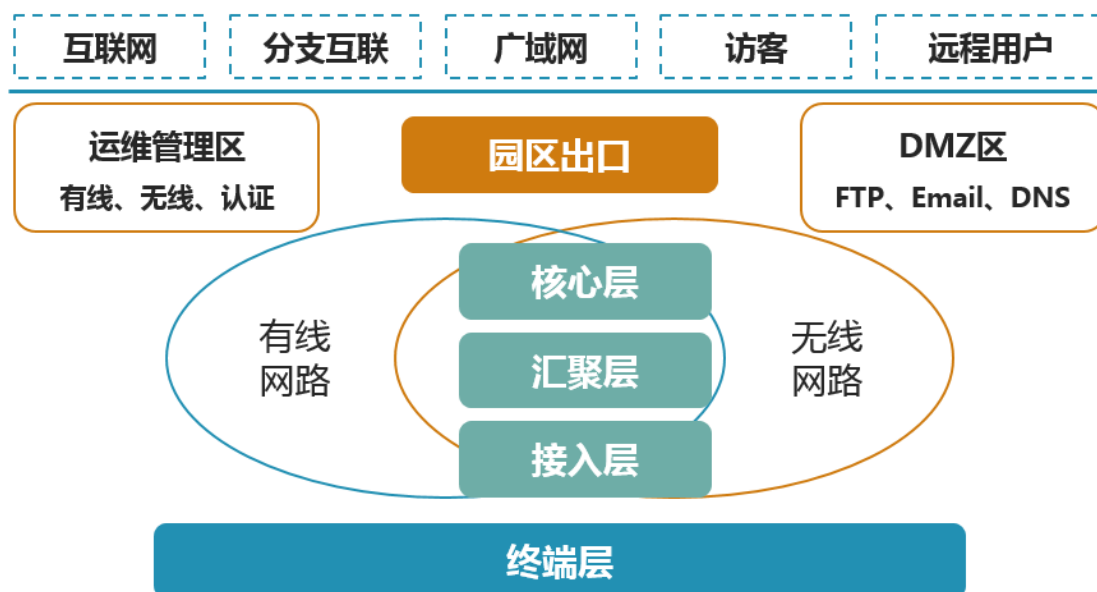
园区网络逻辑结构示
