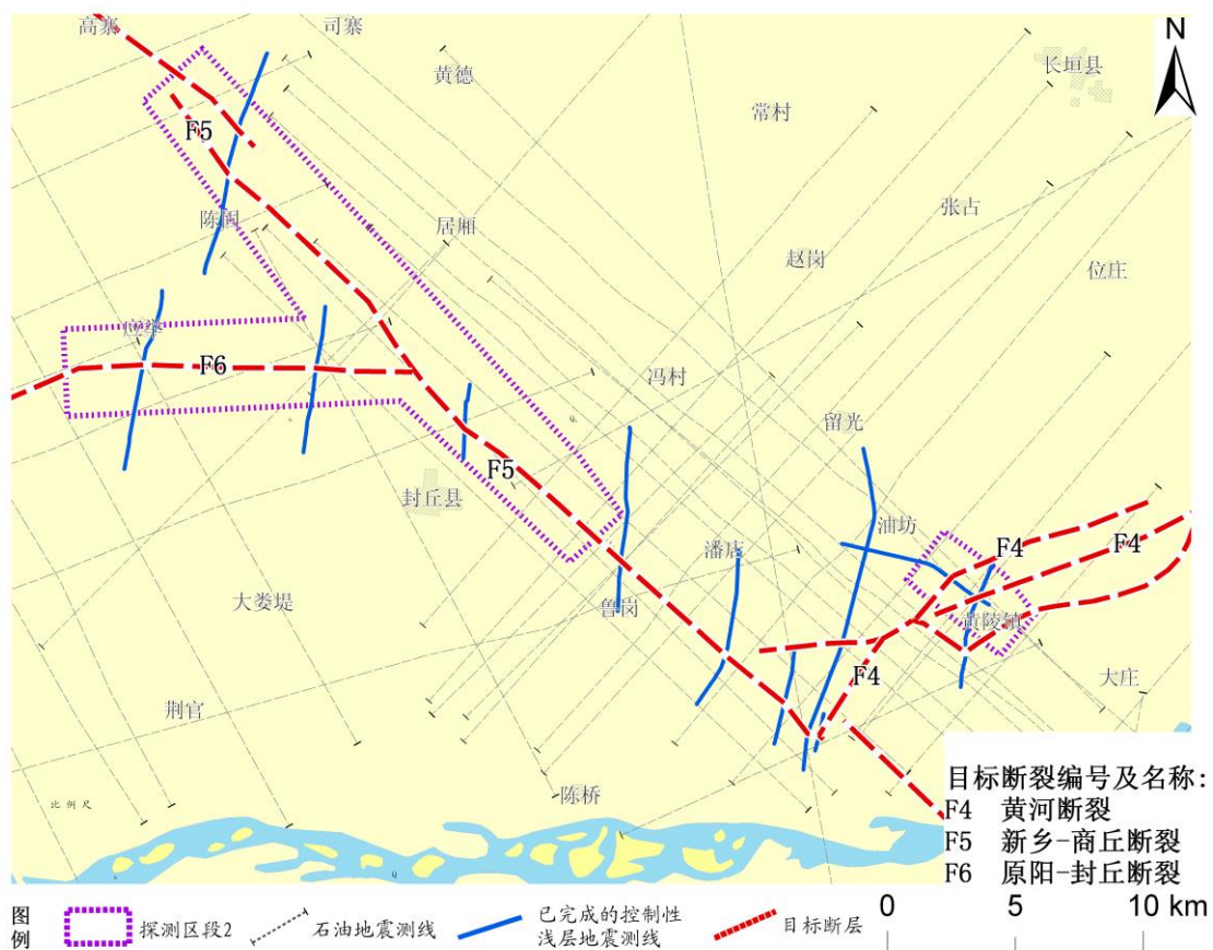
图 7.1-2 封丘地区目标断裂与探测区段分布图
